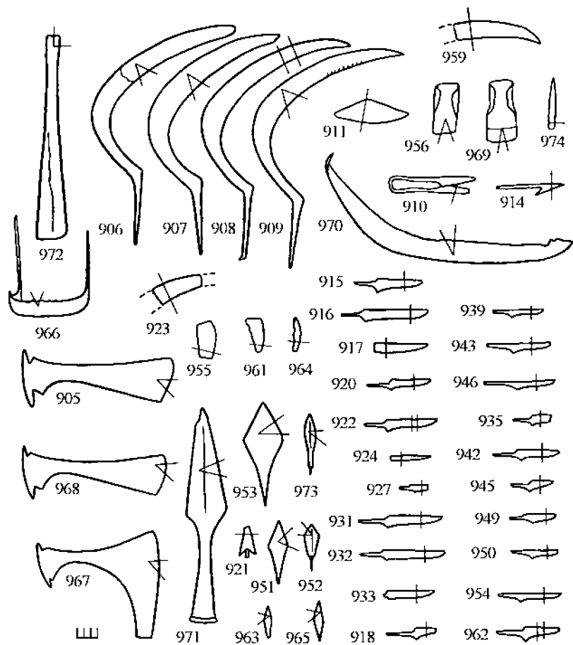
Рис.46. Кузнечная продукция из раскопок Большого Горнальского городища, подвергнутая технологическим исследованиям (по Г.А. Вознесенской) Номера соответствуют номерам анализов
